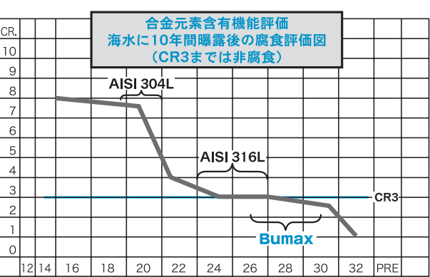
図2 金属材料別腐食試験結果
