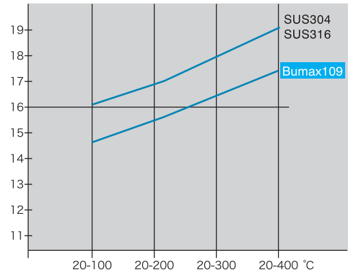
図3 熱膨張係数
