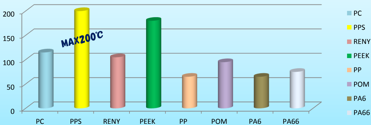
耐熱性比較 (UL認定温度)°C
