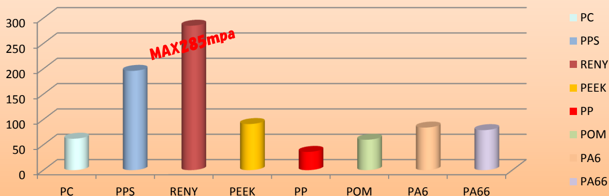
強度比較 (引張り強さ) ASTM D638(mpa)
